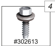
4 #302613 Dichtschraube JA3-6,5x32-E16/2 Sealing screw JA3-6,5x32-E16/2
